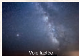
Voie lactée
